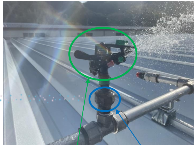
再利用した樹脂製スプリンクラー 427-AGと角度調整用の継手
