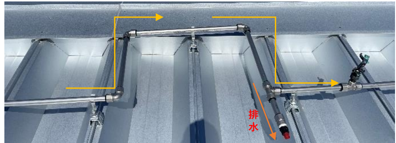
【ステンレスパイプ配管の伸縮対策】 細かな設計が資材の長持ちに繋がります。
